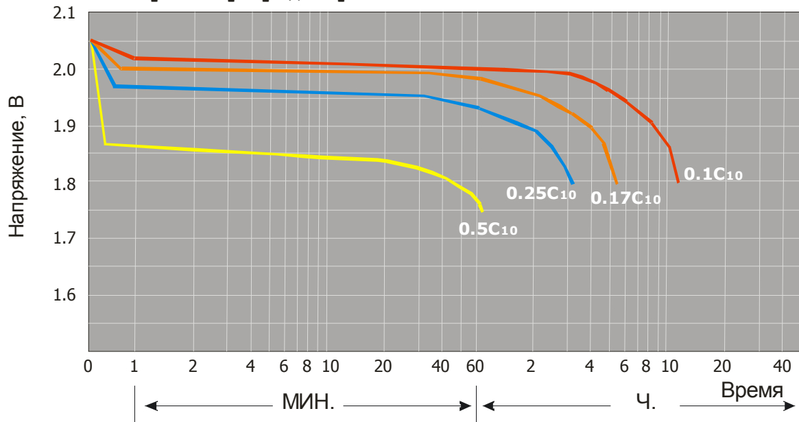
Кривые разряда при 20 °С
