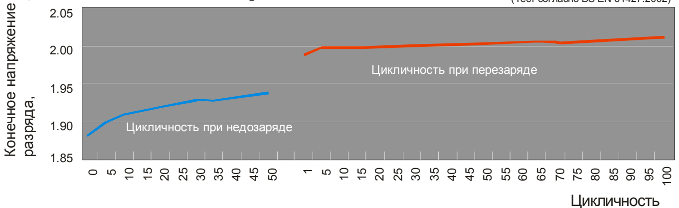
Цикличность батарей
