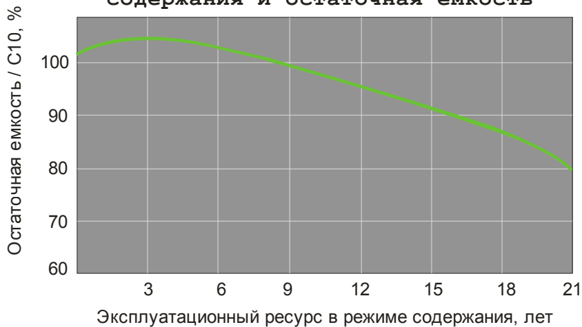
Эксплуатационный ресурс в режиме содержания и остаточная емкость
