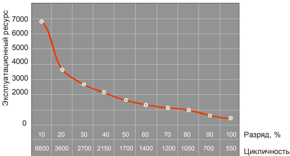
Эксплуатационный ресурс от степени разряда
